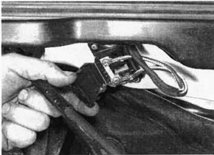
Рис. 3.8. Плавкая вставка цепи питания накаливающей лампы дизельного двигателя (показана одна из первых моделей)
