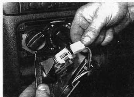
Рис. 11.6,в. ... затем отсоедините электропроводку прикуривателя и снимите панель выключателей
