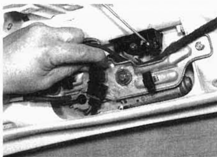
Рис. 15.5,б. ... и разъедините электропроводки от двигателя и освободите электропроводку от хомутов
