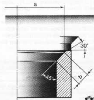
Рис. 4.27. Профиль седла выпускного клапана: a = 32,40 мм; b = 2,4 мм
