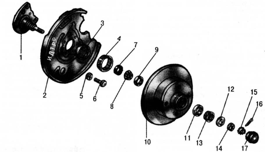
Рис. 6.6. Тормозной диск (ступица) и его детали: 1 – цапфа; 2 – тормозной щит; 3 – кольцо; 4 – венец датчика АБС; 5 – шайба; 6 – болт; 7 – сальник; 8 – внутреннее кольцо внутреннего подшипника; 9 – наружное кольцо внутреннего подшипника; 10 – диск (ступица); 11 – наружное кольцо наружного подшипника; 12 – упорная шайба; 13 – внутреннее кольцо наружного подшипника; 14 – гайка ступицы; 15 – корончатая стопорная шайба; 16 – шплинт; 17 – защитный колпак
