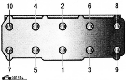
Рис. 4.18. Последовательность затяжки болтов крепления головки блока цилиндров
