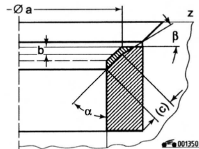
Рис. 4.33. Профиль седла выпускного клапана: Z – привалочная поверхность головки блока цилиндров; a = 33,5 мм; c = 2,0–2,5 мм; α = 45°; β = 30°; γ = 75°
