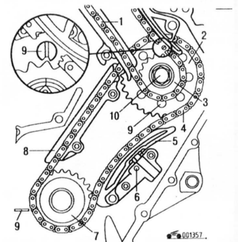
Рис. 4.14. Метка для установки поршня 1-го цилиндра в ВМТ: 1 – цепь привода распределительных валов; 2 – ведомая звездочка промежуточного вала; 3 – ведущая звездочка промежуточного вала; 4 – цепь привода промежуточного вала; 5 – башмак гидронатяжителя цепи привода промежуточного вала; 6 – фиксатор натяжителя цепи привода промежуточного вала; 7 – звездочка коленчатого вала; 8 – успокоитель цепи привода промежуточного вала; 9 – установочные метки; 10 – болт крепления звездочек промежуточного вала
