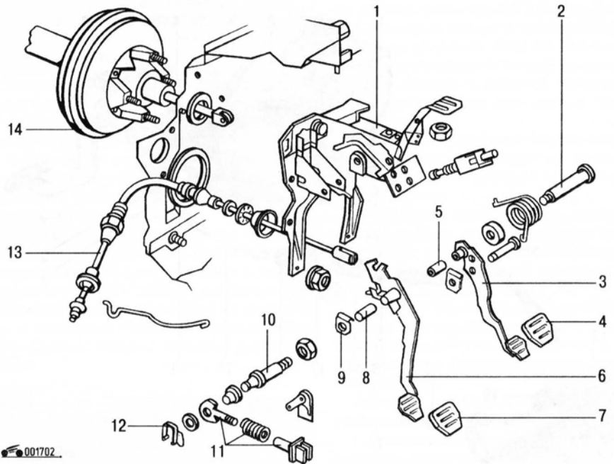
Рис. 5.2. Педаль сцепления с тросовым приводом: 1 – кронштейн педали; 2 – ось педалей сцепления и тормоза; 3 – педаль тормоза; 4, 7 – накладки педалей сцепления и тормоза; 5, 8 – втулки; 6 – педаль сцепления; 9 – пружинный фиксатор; 10 – ось сервомеханизма; 11 – сервомеханизм; 12 – пружинный зажим; 13 – трос сцепления; 14 – вакуумный усилитель тормозов
