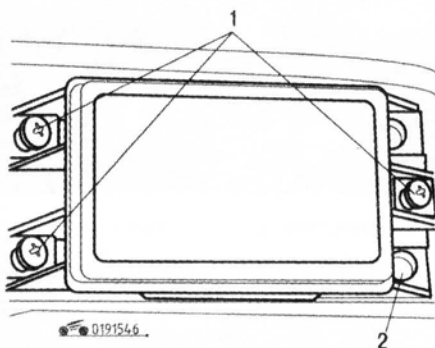
Рис. 9.22. Расположение крепежных элементов противотуманной фары: 1 – винты крепления; 2 – винт регулировки света по вертикали
