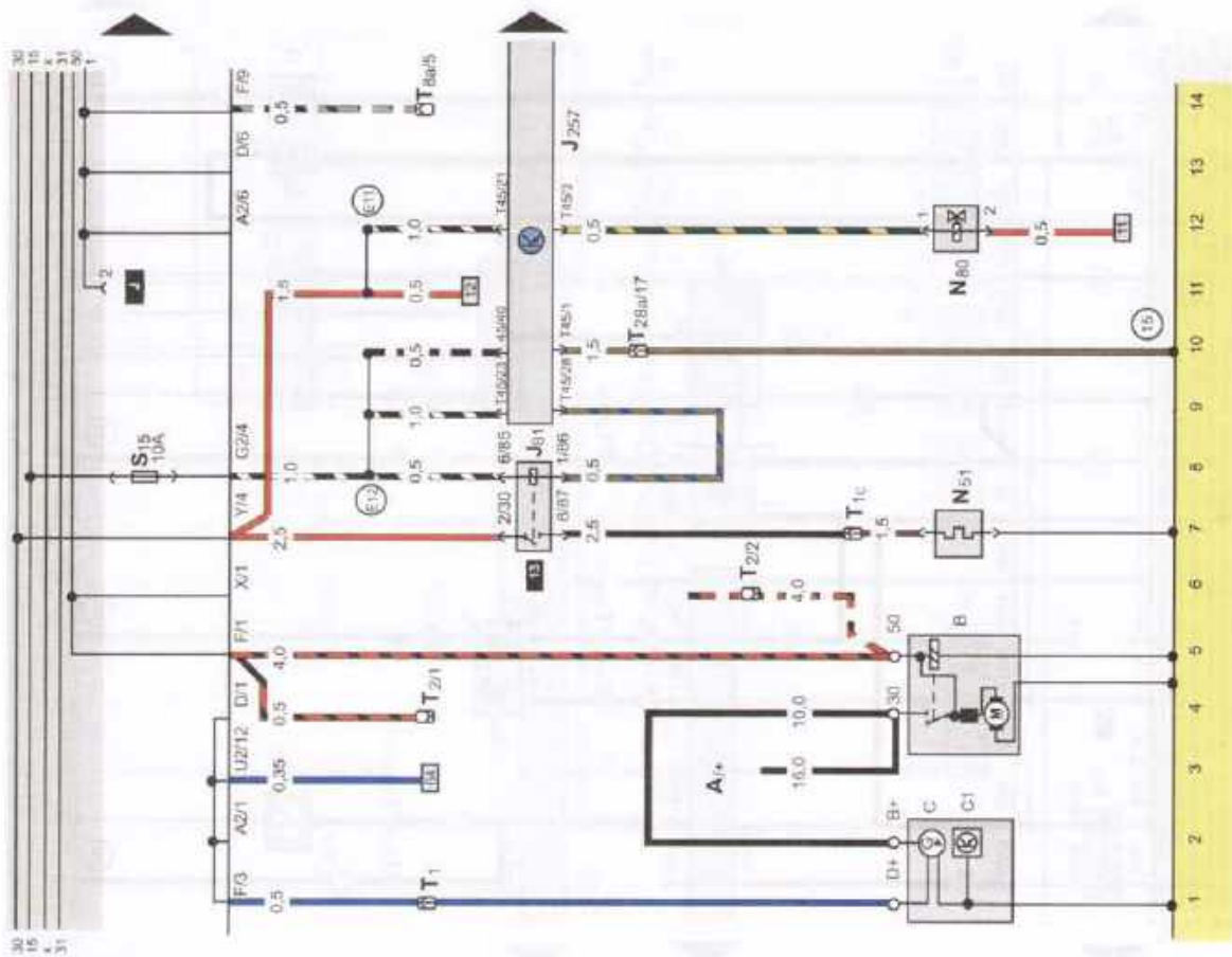
Электрическая схема 48. Система электроснабжения и система пуска двигателя. Двигатели ААМ и АБС с 1994 г.
