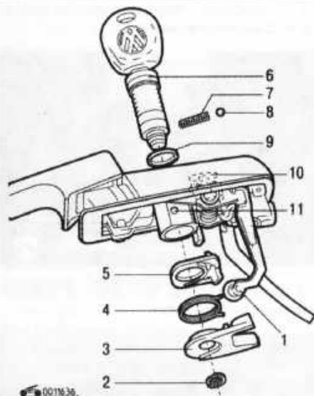
Рис. 10.4. Детали цилиндра замка: 1 – регулировочный болт; 2 – пружинное стопорное кольцо; 3 – рычаг; 4 – пружины; 5 – ограничитель; 6 – цилиндр замка; 8 – шарик; 9 – уплотнительное кольцо; 10 – микропереключатель; 11 – монтажное отверстие
