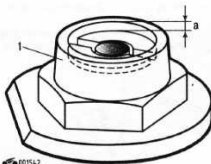
Рис. 4.74. Регулировка стопорного винта плунжера управления: 1 – гайка набивного уплотнения; а = 0,6 мм (расстояние от стопорного винта до торца гайки)
