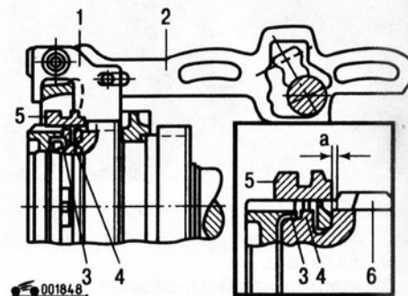
Рис. 5.22. Элементы механизма включения V передачи: 1 – вилка включения V передачи; 2 – рычаг перемещения вилки V передачи; 3 – пружина; 4 – кольцо синхронизатора; 5 – скользящая муфта синхронизатора; 6 – шестерня; а – зазор, равный 1,2 мм
