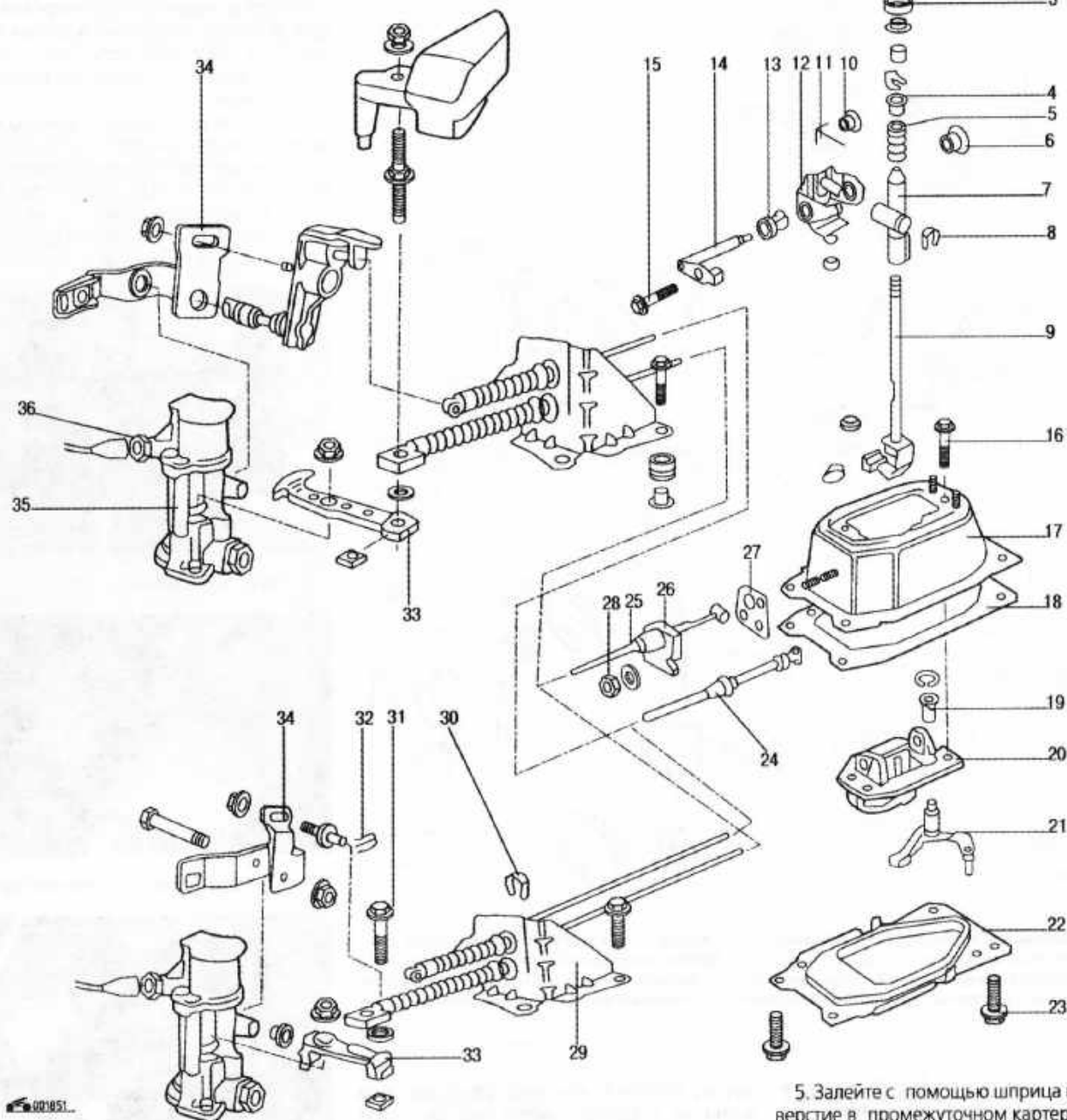
Рис. 5.13. Механизм управления коробкой передач: 1 – рукоятка рычага переключения передач; 2 – защитный кожух рычага; 3 – втулка крепления кожуха рычага; 4, 6, 13, 19 – втулки; 5, 11 – пружины; 7 – направляющая рычага; 8 – пружинное стопорное кольцо; 9 – рычаг переключения передач; 10 – направляющая втулка; 12 – корпус механизма; 14 – штифт; 15, 16, 23 – болты; 17 – корпус рычага переключения передач; 18, 27 – прокладки; 20 – опорная гилита; 21 – рычаг механизма выбора передач; 22 – крышка; 24 – трос предварительного выбора передач; 25 – трос переключения передач; 26 – пластина крепления оболочек тросов к корпусу; 28 – гайка; 29 – кронштейн крепления тросов; 30 – болт крепления троса выбора передач; 31 – болт крепления троса переключения передач; 32 – фигурная пружинная стопорная шайба; 33 – рычаг переключения передач; 34 – рычаг предварительного выбора передач; 35 – механизм выбора передач; 36 – выключатель фонарей заднего хода
