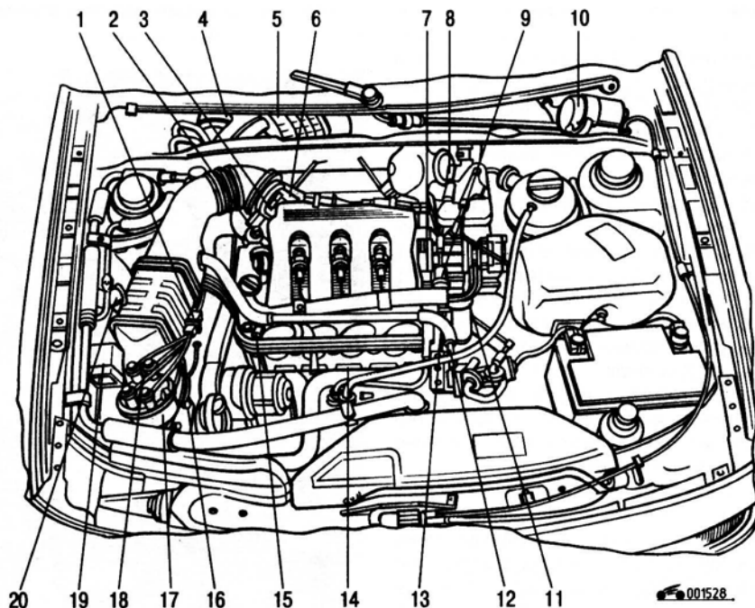
Рис. 4.60. Расположение элементов системы K-Jetronic в моторном отсеке: 1 – датчик давления; 2 – винт регулировки частоты вращения холостого хода; 3 – датчик положения дроссельной заслонки; 4 – коммутатор; 5 – блок управления; 6 – корпус дроссельной заслонки; 7 – распределитель зажигания; 8 – катушка зажигания; 9 – клапан стабилизации холостого хода; 10 – блок управления частотой вращения холостого хода и отключением подачи топлива; 11 – датчик температуры и термовыключатель; 12 – клапан холодного пуска; 13 – клапан подогрева; 14 – сапун картера; 15 – форсунка; 16 – заслонка подогрева поступающего в двигатель воздуха; 17 – распределитель топлива; 18 – винт регулировки СО; 19 – воздушный фильтр; 20 – клапан отключения подачи топлива
