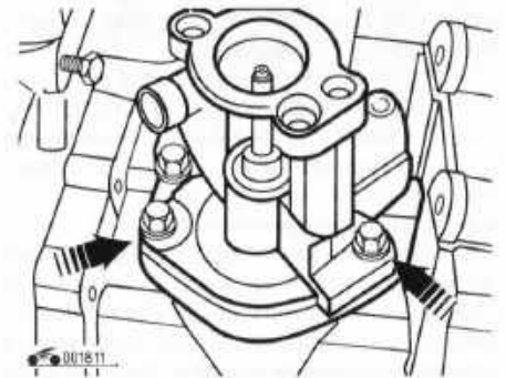
Рис. 5.16. Расположение болтов крепления вала механизма переключения передач
