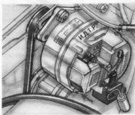
Рис. 9.5. Генератор Valeo
