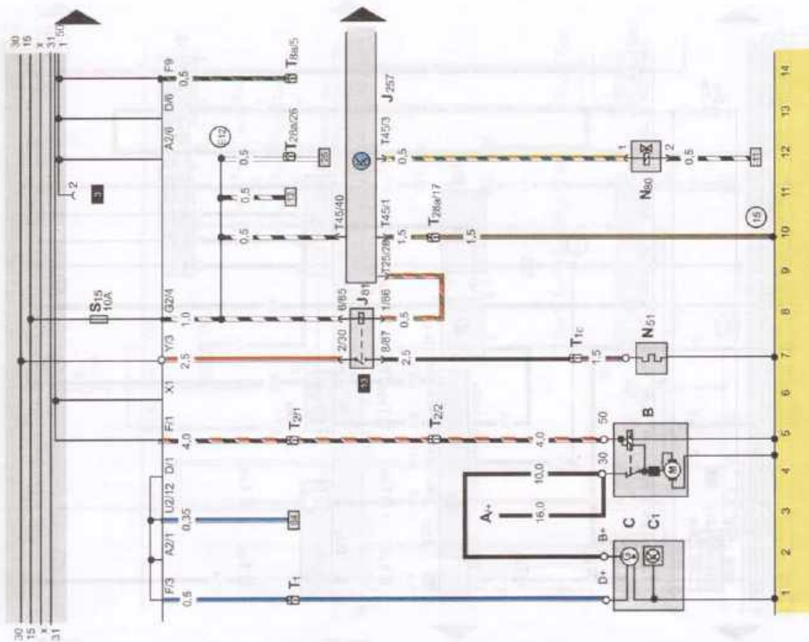
Электрическая схема 51. Система электроснабжения и система пуска двигателя. Двигатель ADZ с 1994 г.
