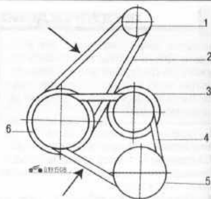
Рис. 4.7. Проверка натяжения ремней привода вспомогательных агрегатов на автомобилях, оборудованных гидроусилителем рулевого управления: 1 – шкив генератора; 2 – ремень привода генератора; 3 – шкив водяного насоса; 4 – ремень привода водяного насоса и насоса гидроусилителя рулевого управления; 5 – шкив насоса гидроусилителя рулевого управления; 6 – шкив коленчатого вала
