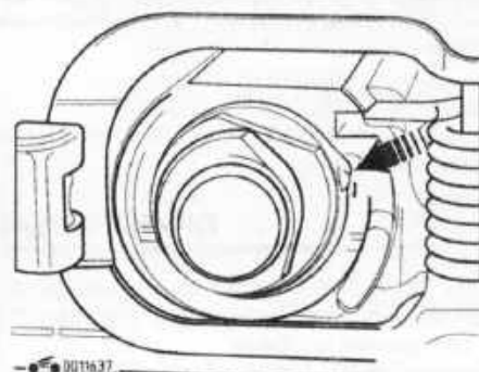
Рис. 10.5. Проверка положения шарика (показан стрелкой) цилиндра замка
