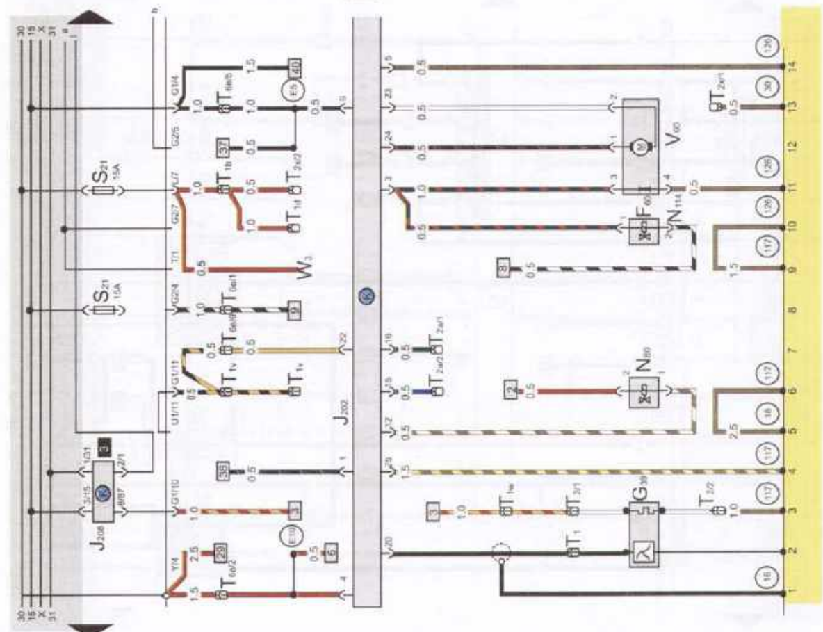
Электроническая схема 34. Система впрыска топлива Mono-Jetronic. Двигатель ЯР с августа 1990 г.
