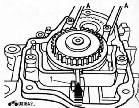
Рис. 5.23. Регулировка положения вилки включения V передачи: А – щупы толщиной 1,2 мм; 1 – болт крепления рычага (стрелкой указано направление оттяжки вилки при регулировке)
