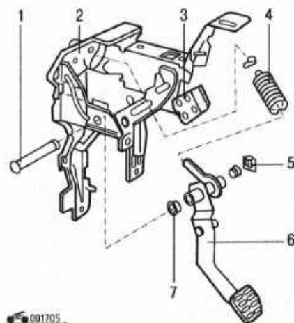
Рис. 5.5. Элементы унифицированного кронштейна педали сцепления: 1 – ось педали; 2 – кронштейн педали; 3 – опора; 4 – сервопружина; 5 – пружинный фиксатор; 6 – педаль сцепления; 7 – втулка
