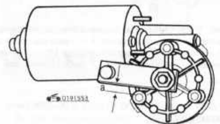
Рис. 9.24. Положение кривошипа на валу моторедуктора. При установке выдержать размер a = 5 мм
