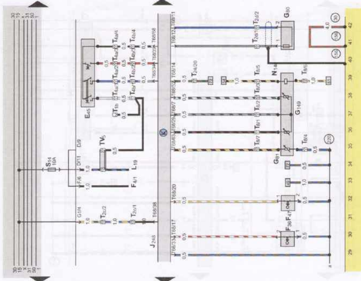
Электрическая схема 60. Система управления дизельным двигателем АГН (продолжение)
