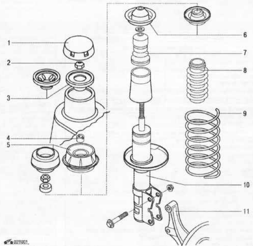
Рис. 6.2. Телескопическая амортизаторная стойка: 1 – защитная крышка; 2 – гайка крепления стойки; 3 – втулка; 4 – шлицевая гайка; 5 – верхняя опора; 6 – верхняя чашка пружины; 7 – буфер сжатия; 8 – защитный чехол; 9 – пружина; 10 – амортизаторная стойка; 11 – поворотный кулак
