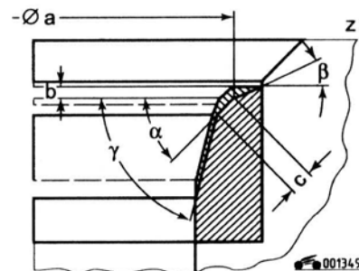
Рис. 4.32. Профиль седла впускного клапана: Z – привалочная поверхность головки блока цилиндров; a = 38,3 мм; c = 1,4–2,0 мм; α = 45°; β = 30°; γ = 75°
