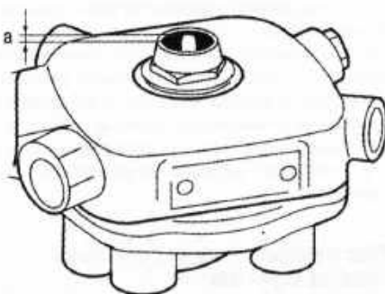
Рис. 4.73. Система впрыска KE-Motronic (регулировка свободного хода распределителя топлива): а = 0,6 мм
