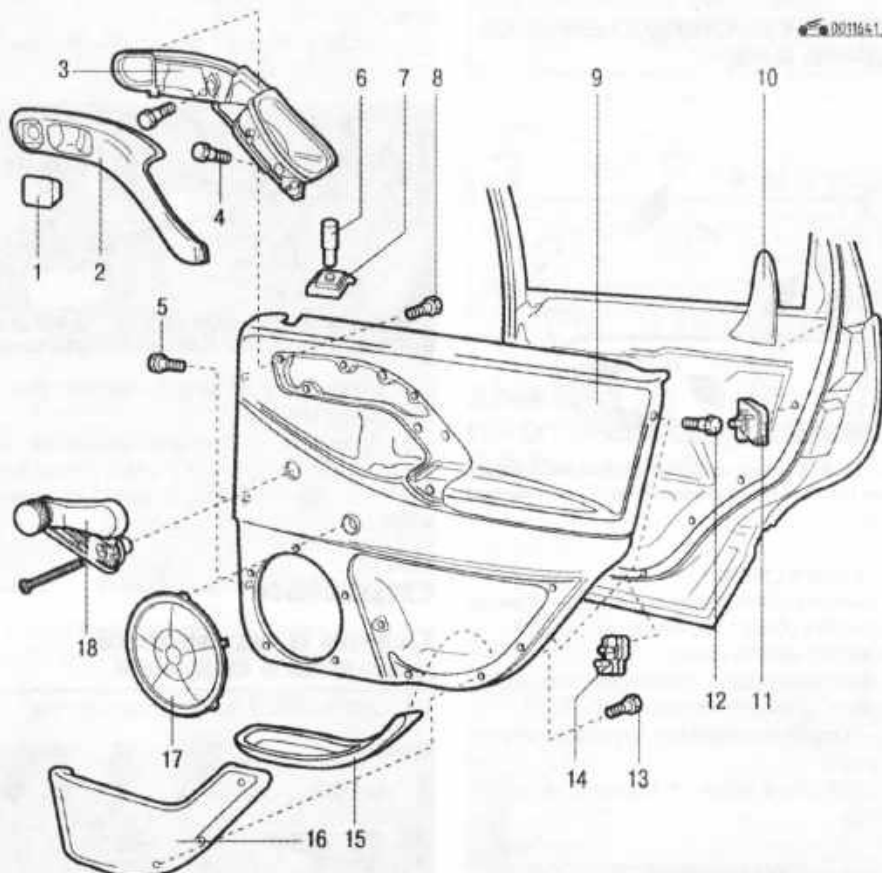
Рис. 10.6. Детали обивки задней двери: 1 – заглушка; 2 – декоративная накладка дверной ручки; 3 – дверная ручка; 4, 5, 8, 12, 13 – винты; 6 – кнопка блокировки дверного замка; 7 – направляющая кнопки блокировки замка; 9 – обивка двери; 10 – декоративная накладка; 11, 14 – скобы; 15 – резиновая отделка; 16 – карман; 17 – решетка динамика аудиосистемы; 18 – ручка стеклоподъемника
