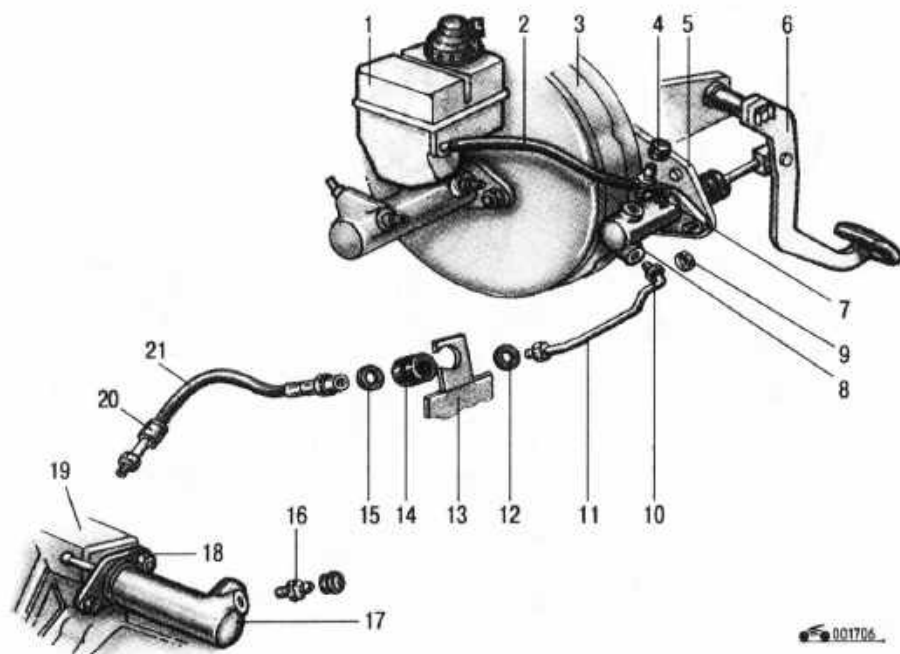
Рис. 5.4. Элементы гидравлического привода выключения сцепления: 1 – бак главного тормозного цилиндра/гидравлического привода выключения сцепления; 2 – шланг подачи жидкости; 3 – вакуумный усилитель тормозов; 4 – защитный колпачок; 5 – кронштейн сервопривода тормозов; 6 – педаль сцепления; 7 – штуцер прокачки главного цилиндра сцепления; 8 – главный цилиндр сцепления; 9 – гайка крепления кронштейна главного цилиндра сцепления; 10 – муфта трубопровода; 11 – трубопровод; 12 – прокладка; 13 – опора; 14 – втулка; 15 – прокладка; 16 – штуцер прокачки рабочего цилиндра сцепления; 17 – рабочий цилиндр сцепления; 18 – гайка крепления рабочего цилиндра; 19 – картер сцепления; 20 – муфта гибкого шланга; 21 – гибкий шланг
