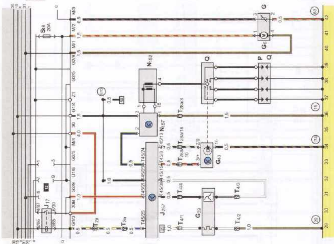
Электрическая схема 53. Система управления двигателем Мопо-Motronic (окончание). Двигатель ADZ с 1994 г.
