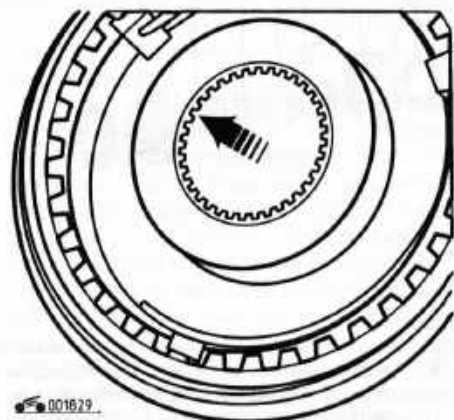
Рис. 5.27. Канавка на внутренней поверхности ступицы синхронизатора III и IV передач должна быть направлена к IV передаче
