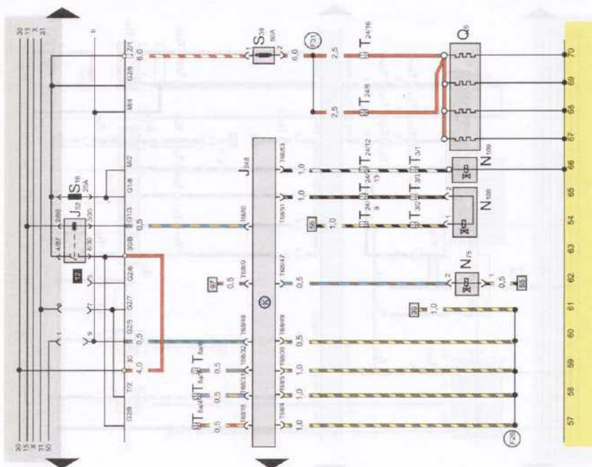
Электрическая схема 62. Система управления дизельным двигателем АГН (продолжение)
