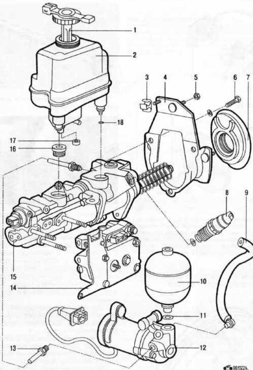
Рис. 8.4. Элементы блока АБС: 1 – пробка; 2 – бачок; 3 – держатель тормозных трубок; 4 – кронштейн; 5 – гайка; 6 – болт; 7 – прокладка; 8 – датчик давления; 9 – соединительный шланг; 10 – гидравлический аккумулятор давления; 11, 18 – уплотнительные кольца; 12 – электрический насос; 13 – тормозная трубка; 14 – блок клапанов; 15 – блок гидравлического усилителя и главный тормозной цилиндр; 16 – соединительная втулка; 17 – втулка
