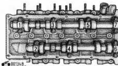
Рис. 4.22. Распределительные валы и крышки их подшипников
