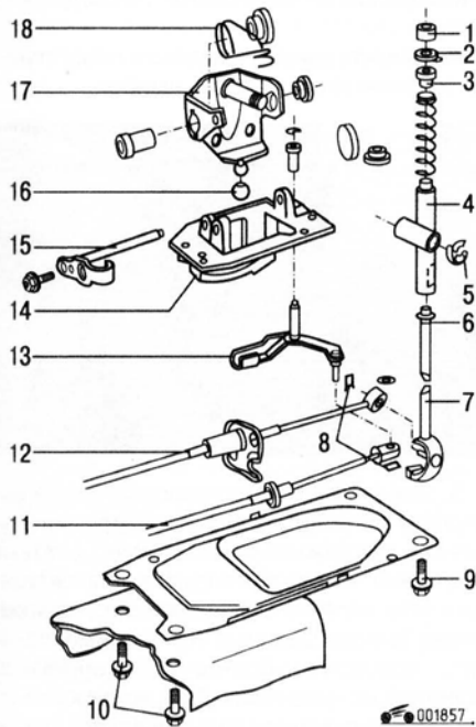
Рис. 5.36. Детали рычага переключения передач: 1 – втулка крепления отделки рычага; 2 – пружинная шайба; 3 – втулка; 4 – направляющая рычага; 5 – стопорное кольцо; 6 – конусная стопорная шайба; 7 – рычаг переключения передач; 8 – пружинные зажимы; 9 – болт; 10 – болты крепления термозащитного экрана; 11 – трос предварительного выбора передач; 12 – трос переключения передач; 13 – рычаг механизма предварительного выбора передач; 14 – опорная пластина; 15 – направляющий штифт; 16 – колпачок; 17 – корпус механизма выбора передач; 18 – пружина
