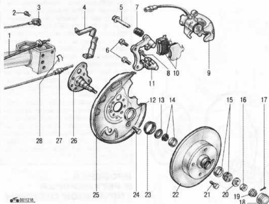
Рис. 8.5. Дисковый тормозной механизм заднего колеса: 1 – трубопровод; 2, 8, 21, 24 – болты; 3 – датчик ABS; 4 – кронштейн; 5 – направляющий штифт; 6 – болты крепления направляющей колодок; 7 – защитный чехол; 9 – суппорт; 10 – тормозные колодки; 11 – направляющая колодок; 12, 13 – уплотнительные кольца; 14 – внутренний подшипник; 15 – наружный подшипник; 16 – гайка; 17 – шплинт; 18 – колпачок; 19 – корончатая стопорная шайба; 20 – упорная шайба; 22 – тормозной диск; 23 – ротор датчика ABS; 25 – защитный кожух; 26 – цапфа; 27 – трос стояночного тормоза; 28 – пружинный зажим
