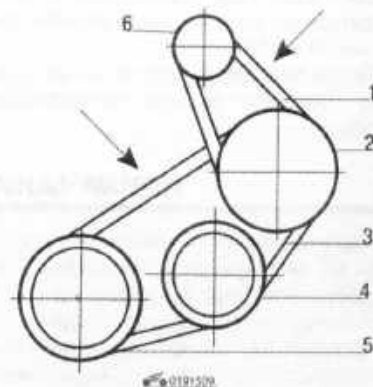
Рис. 4.8. Проверка натяжения ремней привода вспомогательных агрегатов на автомобилях, оборудованных системой кондиционирования: 1 – ремень привода генератора; 2 – шкив компрессора кондиционера; 3 – ремень привода водяного насоса и компрессора кондиционера; 4 – шкив водяного насоса; 5 – шкив коленчатого вала; 6 – шкив генератора
