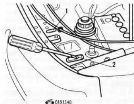
Рис. 9.16. Регулировка потока левой фары на автомобилях с кузовом B3: 1 - в вертикальной плоскости; 2 - в горизонтальной плоскости
