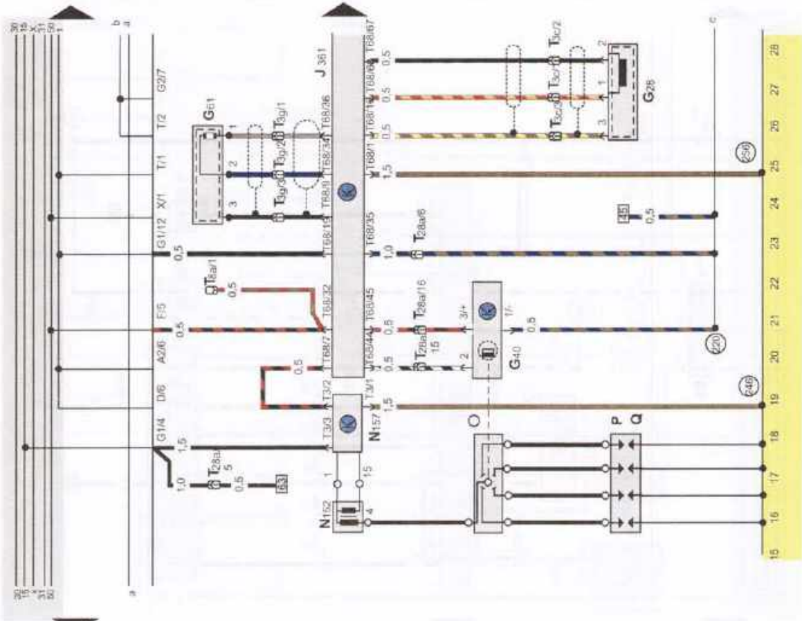
Электрическая схема 44. Система управления двигателем Simos. Все модели с 1994 г.
