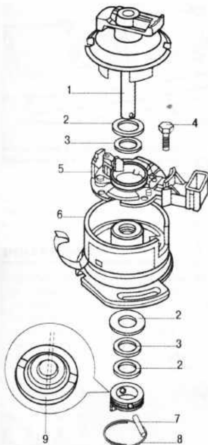
Рис. 9.13. Распределитель систем зажигания FI и KE-Motronic: 1 – вал в сборе с бегунком и стальным экраном с прорезями; 2 – стальная шайба; 3 – пластмассовая шайба; 4 – винт; 5 – датчик Холла; 6 – корпус распределителя; 7 – штифт; 8 – стопорное кольцо; 9 – муфта привода
