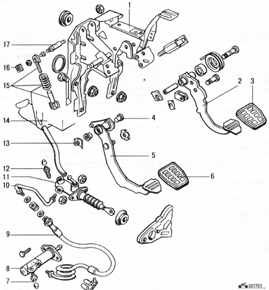
Рис. 5.3. Педаль сцепления с гидравлическим приводом: 1 – кронштейн педали; 2 – педаль тормоза; 3, 6 – накладки педалей сцепления и тормоза; 4 – втулка; 5 – педаль сцепления; 7 – штуцер прокачки рабочего цилиндра сцепления; 8 – рабочий цилиндр сцепления; 9 – гибкий шланг; 10 – трубопровод; 11 – главный цилиндр сцепления; 12 – штуцер прокачки главного цилиндра сцепления; 13 – пружинный фиксатор; 14 – бачок гидравлического привода выключения сцепления/главного тормозного цилиндра; 15 – сервомеханизм; 16 – пружинный фиксатор; 17 – ось сервомеханизма
