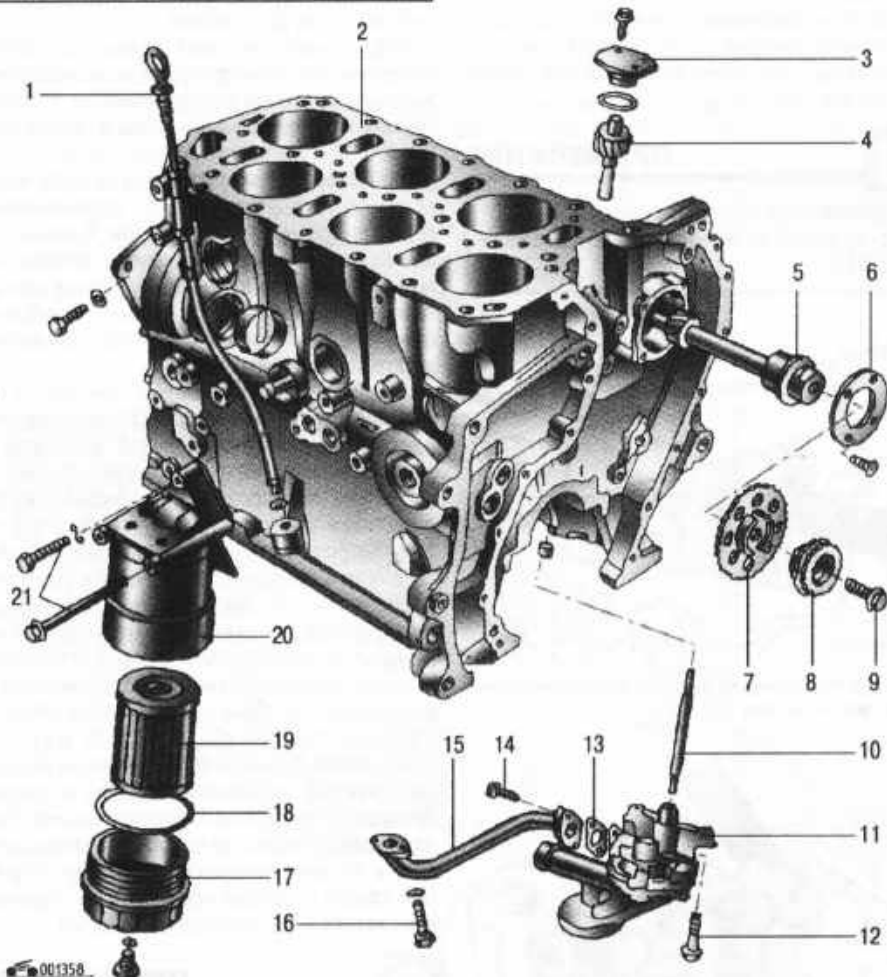
Рис. 4.44. Масляный насос и масляный фильтр: 1 — масляный шуп; 2 — блок цилиндров; 3 — крышка вала привода масляного насоса; 4 — шестерня привода масляного насоса; 5 — промежуточный вал; 6 — крышка промежуточного вала; 7 — ведомая звездочка промежуточного вала; 8 — ведущая звездочка промежуточного вала; 9 — болт крепления звездочек промежуточного вала; 10 — вал привода масляного насоса; 11 — масляный насос; 12 — болт крепления масляного насоса; 13 — прокладка маслоприемной трубы; 14, 16 — болты крепления маслоприемной трубы; 15 — маслоприемная труба; 17 — крышка масляного фильтра; 18 — уплотнительное кольцо; 19 — масляный фильтр; 20 — корпус масляного фильтра; 21 — болты крепления корпуса масляного фильтра
