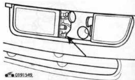
Рис. 9.18. Расположение винта регулировки света противотуманной фары в вертикальной плоскости
