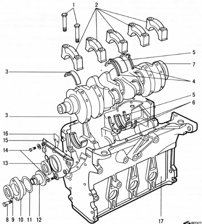
Рис. 4.3. Блок цилиндров, коленчатый и промежуточный валы: 1 – болты крепления крышки коренного подшипника коленчатого вала; 2 – крышка коренного подшипника коленчатого вала; 3 – вкладыш коренного подшипника коленчатого вала; 4, 6 – упорные полукольца; 5 – вкладыш центрального (упорного) коренного подшипника коленчатого вала; 7 – коленчатый вал; 8 – болт крепления крышки промежуточного вала; 9 – сальник промежуточного вала; 10 – крышка промежуточного вала; 11 – уплотнительное кольцо промежуточного вала; 12 – промежуточный вал; 13 – передний сальник коленчатого вала; 14 – болты крепления передней крышки коленчатого вала; 15 – передняя крышка коленчатого вала; 16 – прокладка передней крышки коленчатого вала; 17 – блок цилиндров
