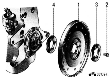
Рис. 4.16. Ведущий диск: 1 – ведущий диск; 2 – болт крепления ведущего диска; 3 – прижимная пластина; 4 – регулировочная шайба
