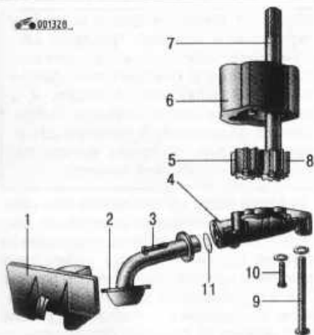
Рис. 4.43. Масляный насос четырехцилиндрового двигателя: 1 — перегородка; 2 — маслоприемник; 3 — болт крепления маслоприемника; 4 — крышка масляного насоса; 5 — ведомая шестерня; 6 — корпус масляного насоса; 7 — вал привода масляного насоса; 8 — ведущая шестерня; 9 — болт крепления масляного насоса; 10 — болт крепления крышки масляного насоса; 11 — уплотнительное кольцо маслоприемника
