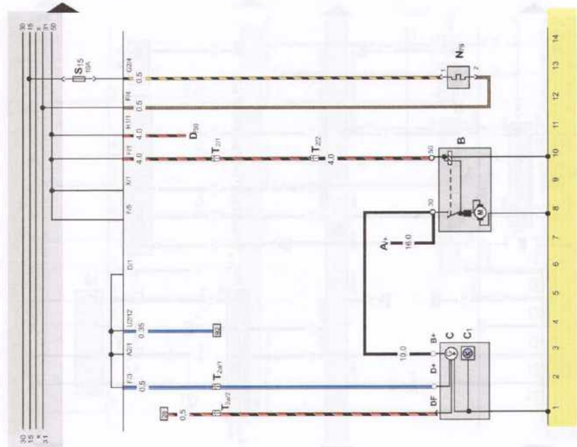
Электрическая схема 58. Система электроснабжения и система пуска дизельного двигателя AFN
