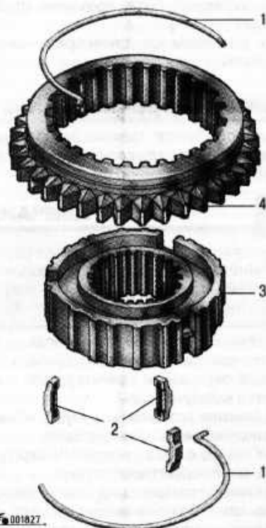
Рис. 5.30. Синхронизатор I и II передач: 1 — пружина; 2 — сухари; 3 — ступица синхронизатора; 4 — скользящая муфта
