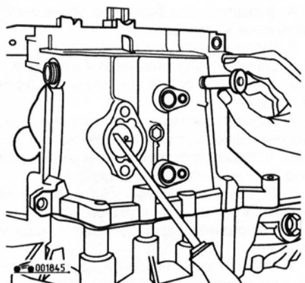
Рис. 5.20. Выравнивание осей вилок с помощью отвертки и цапфы
