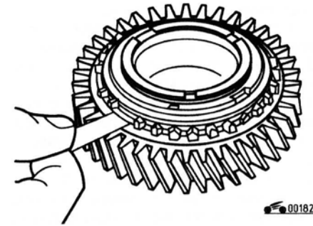
Рис. 5.26. Проверка внешнего кольца синхронизатора II передачи
