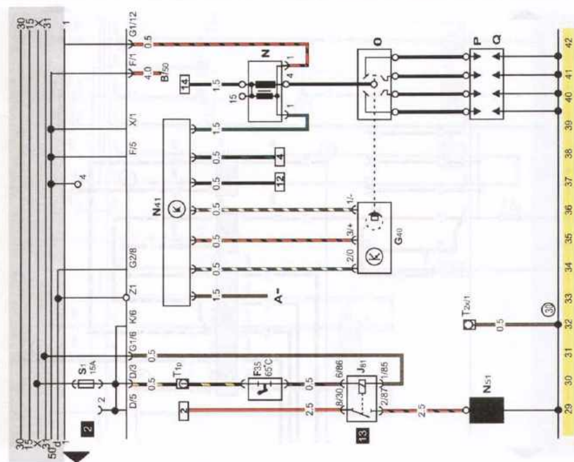
Электрическая схема 25. Система зажигания TSI-N карбюраторных двигателей и двигателей с системой впрыска Mono-Jetronic. Все модели до 1994 г.
