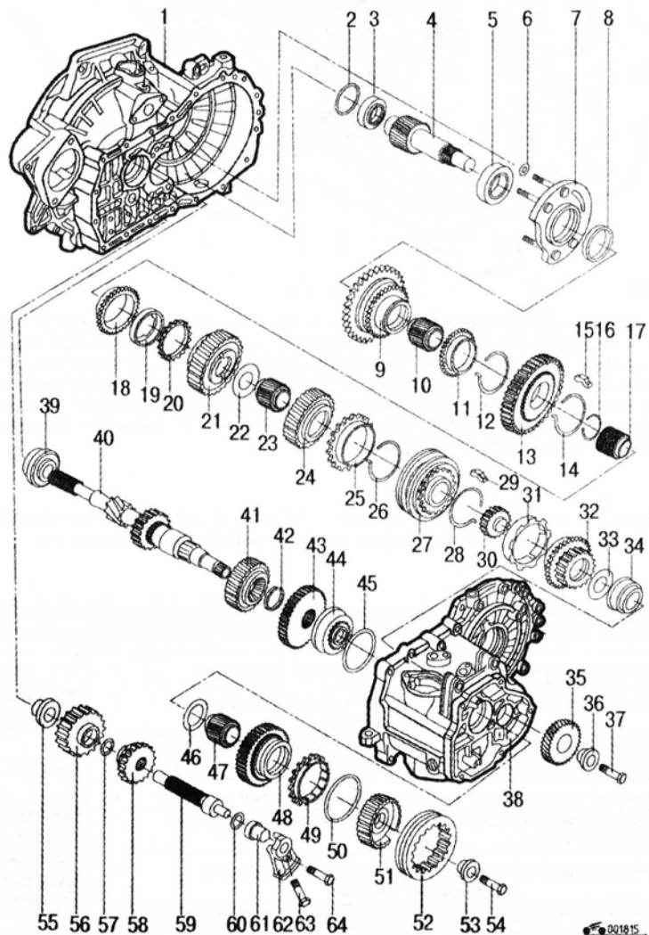
Рис. 5.11. Валы и шестерни пятиступенчатой коробки передач: 1 – картер сцепления; 2 – регулировочная шайба; 3 – конический подшипник (малый); 4 – вторичный вал; 5 – конический подшипник (большой); 6 – шайба круглого сечения; 7 – опора подшипника; 8, 22, 33, 46, 60 – упорные шайбы; 9 – шестерня I передачи; 10, 23, 30, 47 – игольчатые подшипники; 11, 18, 25, 31, 49 – кольца синхронизаторов; 12, 14, 26, 28 – пружины; 13, 15, 29, 27 – синхронизаторы; 16, 17 – стопорные кольца игольчатого подшипника; 19 – внешнее кольцо синхронизатора; 20 – внутреннее кольцо синхронизатора; 21 – шестерня II передачи; 24 – шестерня III передачи; 32 – шестерня IV передачи; 34, 36, 53, 55, 61 – втулки; 35 – шестерня V передачи; 37, 54 – болты М8х26; 38 – картер коробки передач; 39 – роликовый подшипник; 40 – первичный вал; 41 – шестерня I передачи; 42 – стопорное кольцо; 43 – шестерня IV передачи; 44 – роликовый подшипник; 45 – регулировочное кольцо; 48 – шестерня V передачи; 50 – пружина; 51 – ступица синхронизатора; 52 – скользящая муфта синхронизатора; 56 – промежуточная шестерня; 57 – стопорное кольцо; 58 – шестерня передачи заднего хода; 59 – вал шестерни передачи заднего хода; 62 – держатель вала заднего хода; 63 – винт продольного крепления держателя; 64 – винт поперечного крепления держателя
