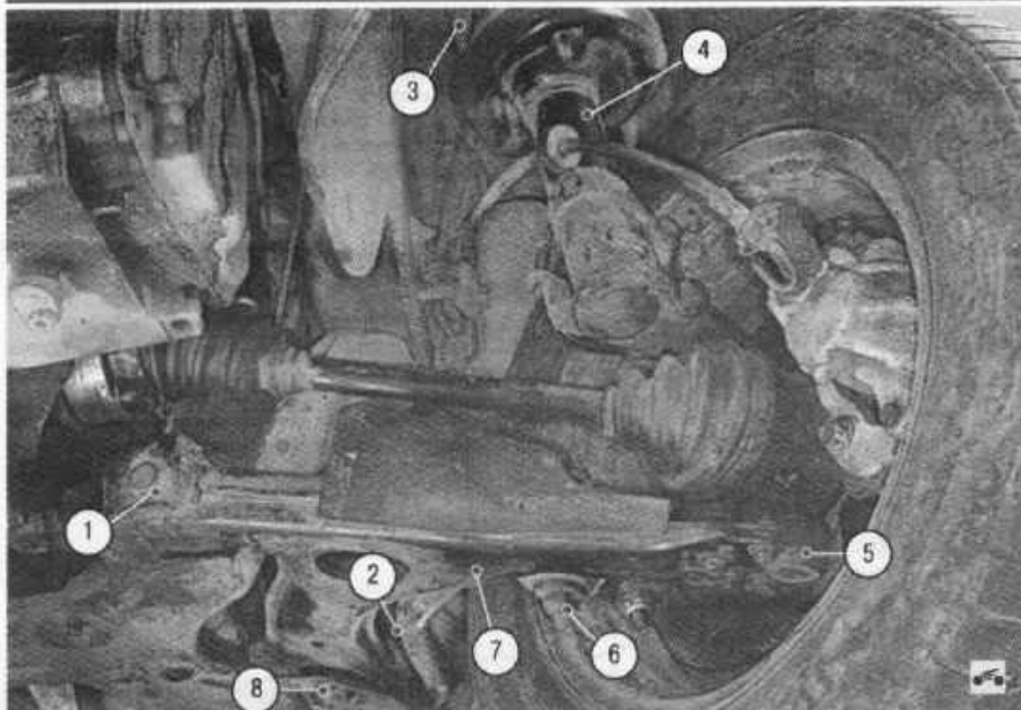
6. Расположение элементов передней подвески на автомобиле: 1 – передняя опора (сайлентблок) рычага передней подвески; 2 – штанга стабилизатора поперечной устойчивости; 3 – пружина передней подвески; 4 – телескопическая стойка; 5 – шаровая опора стойки; 6 – стойка стабилизатора поперечной устойчивости; 7 – рычаг передней подвески; 8 – задняя опора (резиновая втулка) рычага передней подвески
