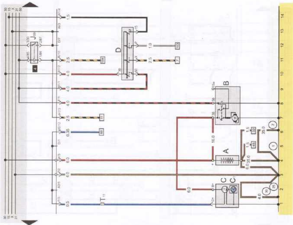
Электрическая схема 32. Система электроснабжения и система пуска двигателя. Двигатели РГ, РВ, РР и 2Е
