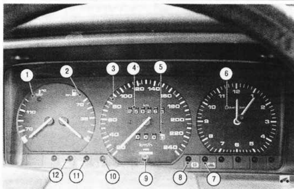
Рис. 1.7. Комбинация приборов
