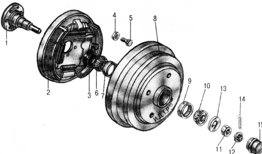
Рис. 6.5. Тормозной барабан (ступица) и его детали: 1 – цапфа; 2 – тормозной механизм; 3 – сальник; 4 – шайба; 5 – болт; 6 – внутреннее кольцо внутреннего подшипника; 7 – наружное кольцо внутреннего подшипника; 8 – барабан (ступица); 9 – наружное кольцо наружного подшипника; 10 – внутреннее кольцо наружного подшипника; 11 – гайка ступицы; 12 – корончатая стопорная шайба; 13 – упорная шайба; 14 – шплинт; 15 – защитный колпак
