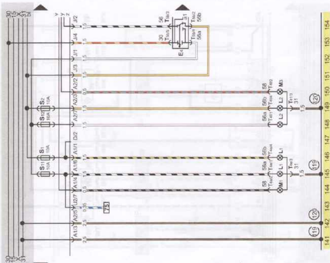
Электрическая схема 11. Фары и габаритное освещение
