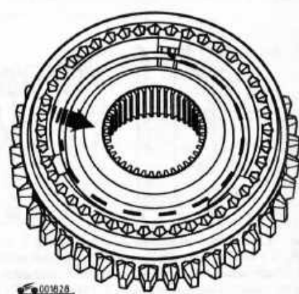
Рис. 5.31. При установке синхронизатора I и II передач более широкий буртик должен быть направлен к шестерне I передачи
