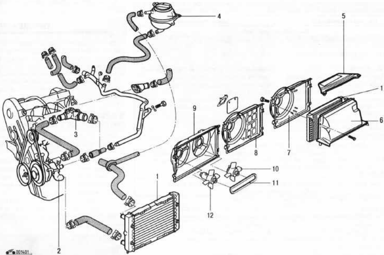
Рис. 4.47. Система охлаждения двигателя SOHC: 1 – радиатор; 2 – водяной насос; 3 – соединительный патрубок; 4 – расширительный бачок; 5 – верхний защитный кожух; 6 – воздушнонаправляющий кожух; 7 – кожух вентилятора (EZ); 8 – кожух вентилятора (PB, RP); 9 – кожух вентиляторов; 10 – дополнительный вентилятор; 11 – приводной ремень; 12 – электрический вентилятор
