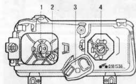
Рис. 9.19. Элементы фары автомобиля с кузовом B4: 1 - лампа ближнего света; 2 - лампа габаритного света; 3 - моторедуктор корректора света фар; 4 - лампа дальнего света
