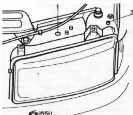
Рис. 9.17. Регулировка потока левой фары на автомобилях с кузовом B4: 1 - в вертикальной плоскости; 2 - в горизонтальной плоскости
