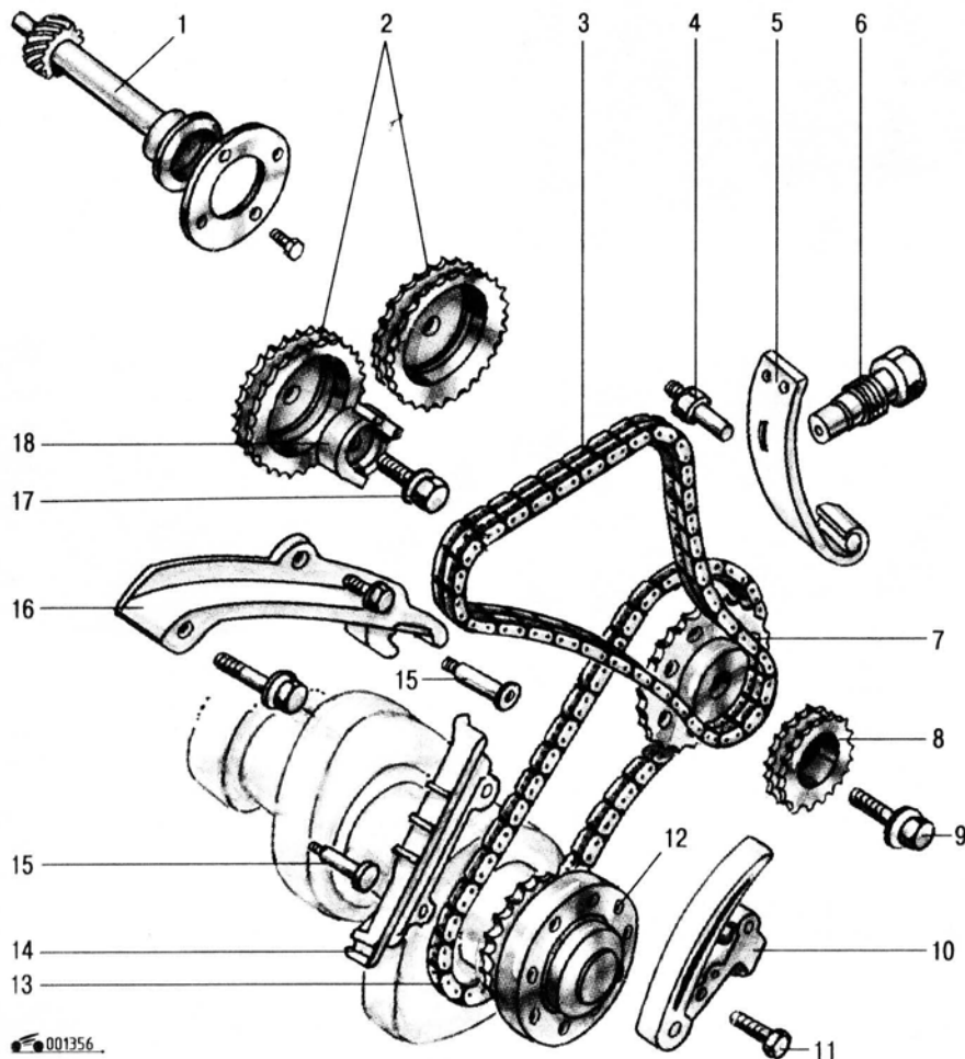
Рис. 4.15. Привод газораспределительного механизма: 1 – промежуточный вал; 2 – звездочки распределительных валов; 3 – цепь привода распределительных валов; 4 – ось башмака натяжителя цепи привода распределительных валов; 5 – башмак натяжителя цепи привода распределительных валов; 6 – болт регулировки натяжения цепи привода распределительных валов; 7 – ведомая звездочка промежуточного вала; 8 – ведущая звездочка промежуточного вала; 9 – болт крепления звездочек промежуточного вала; 10 – гидронатяжитель цепи привода промежуточного вала; 11 – болт крепления натяжителя цепи привода промежуточного вала; 12 – коленчатый вал; 13 – цепь привода промежуточного вала; 14 – успокоитель цепи привода промежуточного вала; 15 – пальцы успокоителя цепи привода промежуточного вала; 16 – успокоитель цепи привода распределительных валов; 17 – болт крепления муфты привода распределителя зажигания и звездочки распределительного вала; 18 – муфта привода распределителя зажигания
