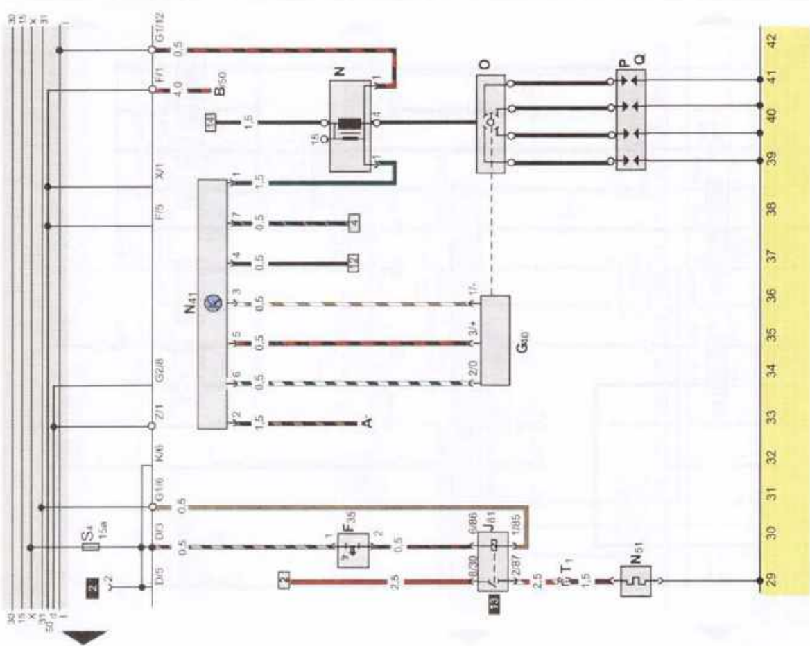
Электрическая схема 36. Система зажигания и подогрев впускного коллектора. Двигатель ЯР с августа 1990 г.
