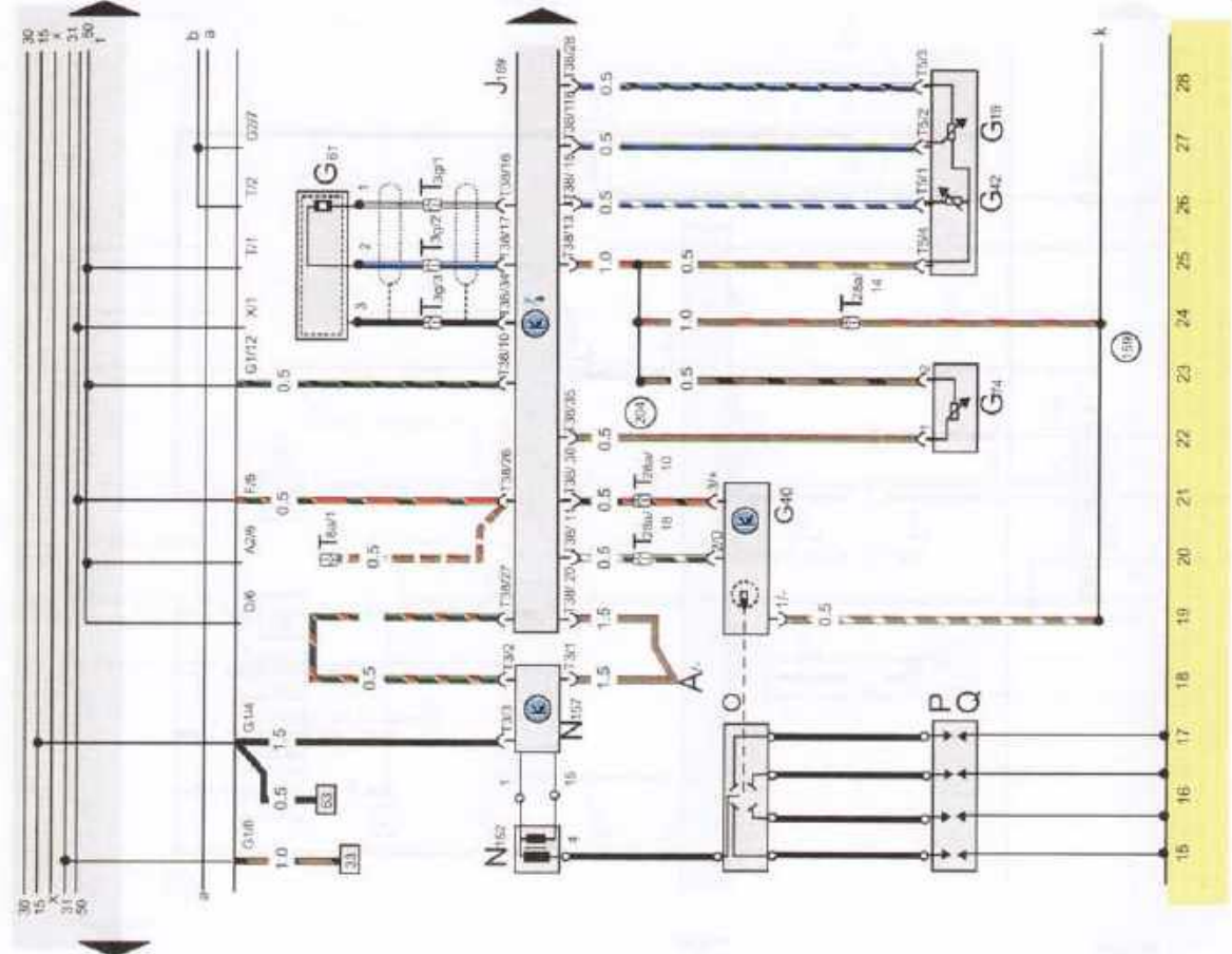
Электрическая схема 40. Система управления двигателем Digifant. Двигатель 2Е с 1994 г.
